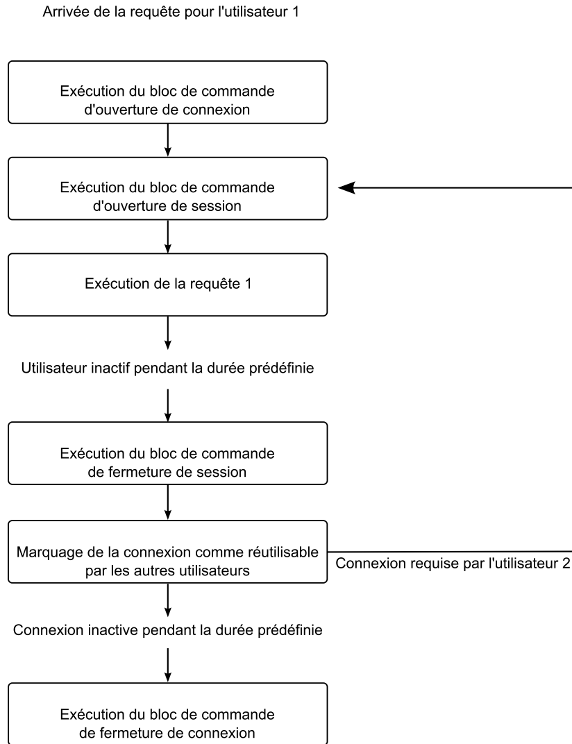
Figure 5. Exemple - Interaction entre des blocs de commande
